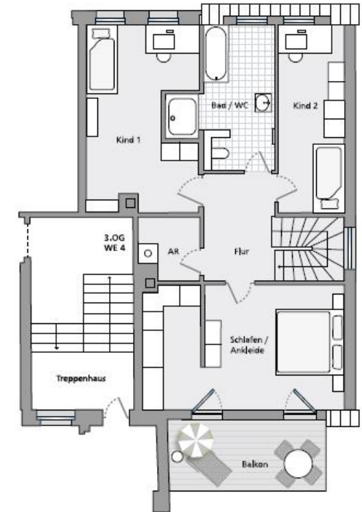
3. Obergeschoss
